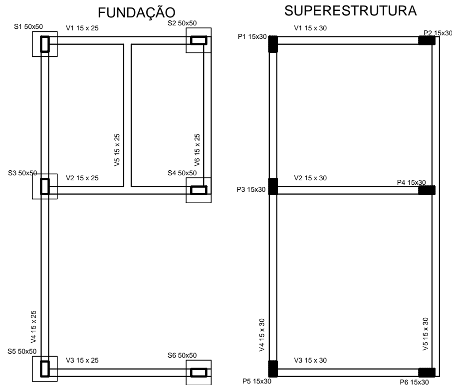
Detalhe fundação ESCALA 1/75
