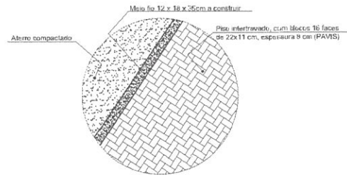
○ Detalhe calçamento Escala 1/50
