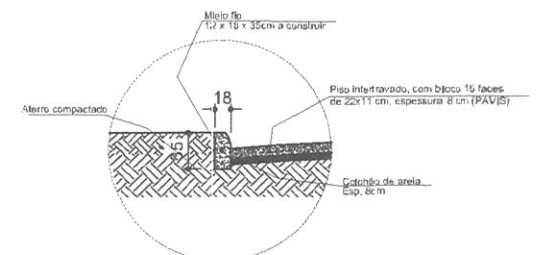
⊙ Detalhe calçamento Escala 1/50
