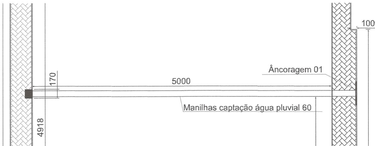
○ Detalhe drenagem Escala 1/50
