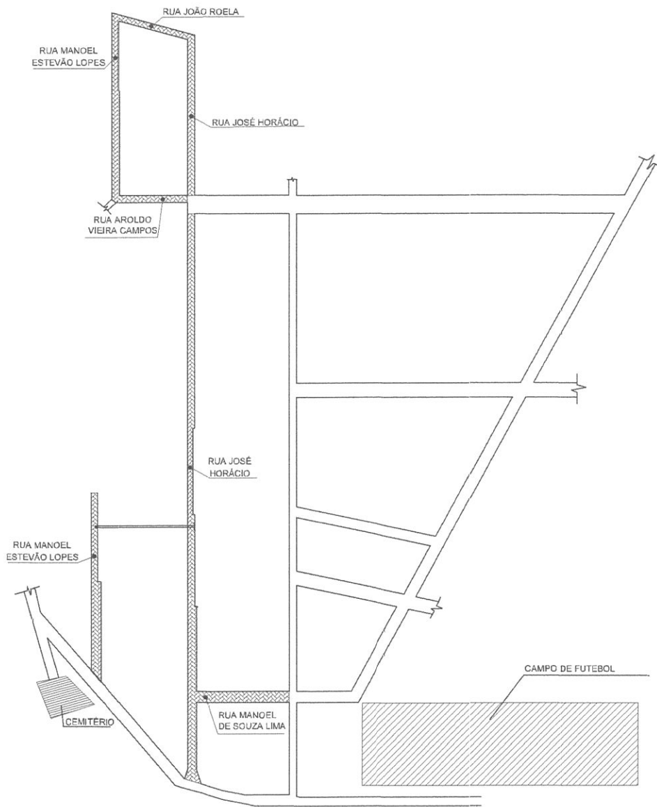
⊙ Detalhe calçamento Escala 1/200
