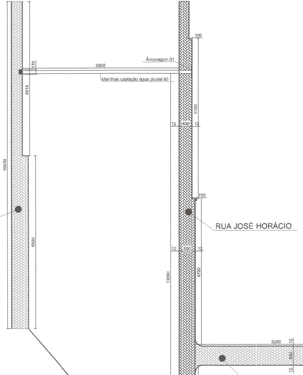
⊕ Detalhe rua Escala 1/50
