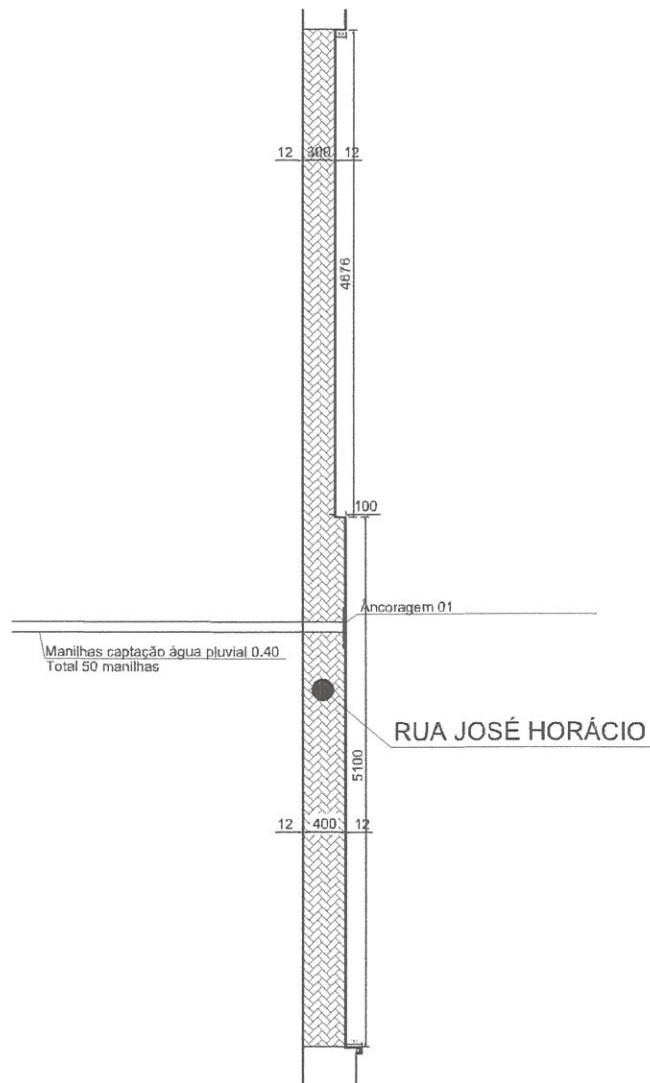
○ Detalhe rua Escala 1/50
