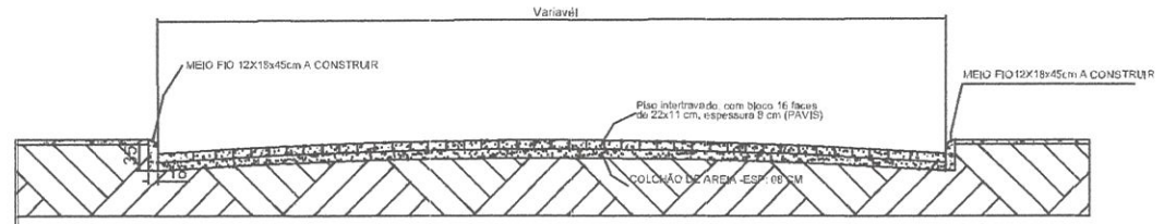
○ Detalhe calçamento Sem escala
