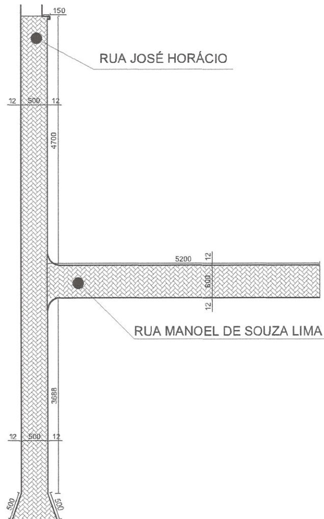
○ Detalhe rua Escala 1/50
