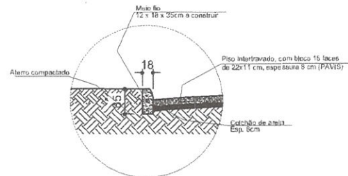
○ Detalhe calçamento Escala 1/50
